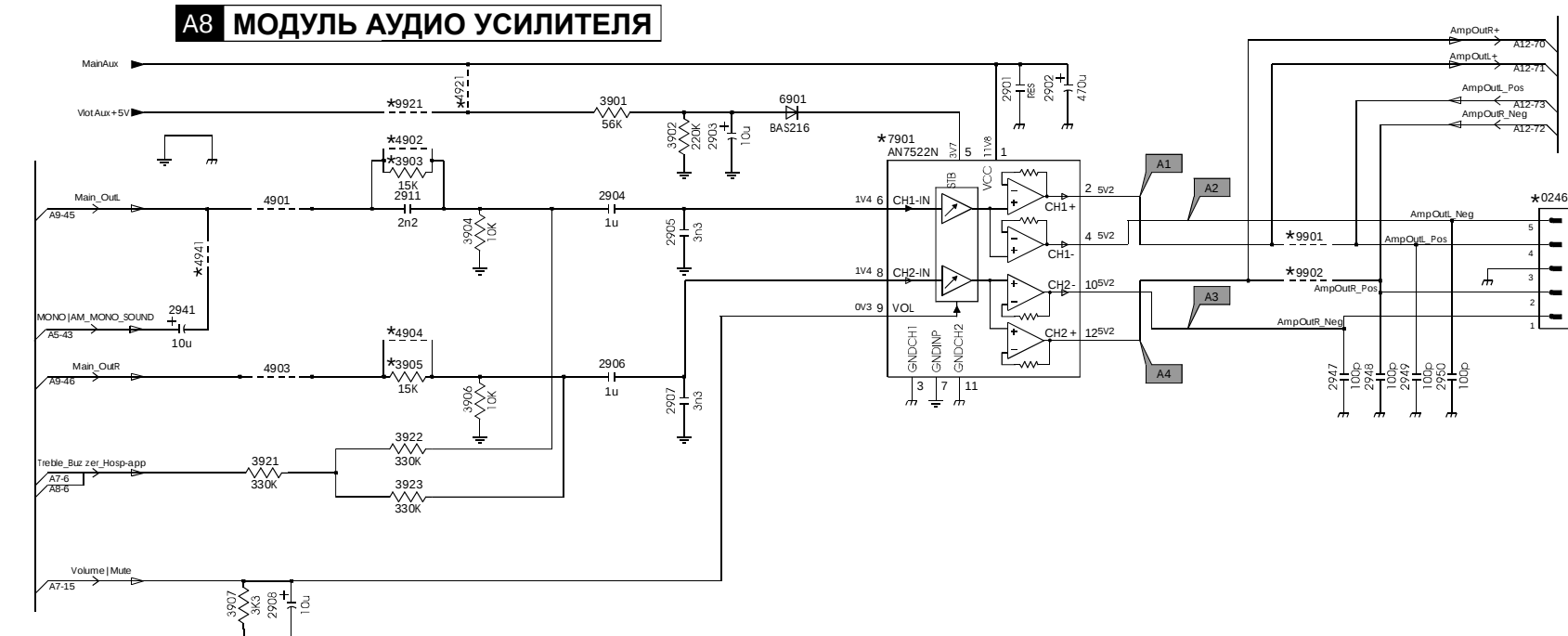
A8 МОДУЛЬ АУДИО УСИЛИТЕЛЯ
